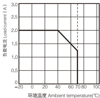
负载电流-环境温度 Load current- Ambient temperature
